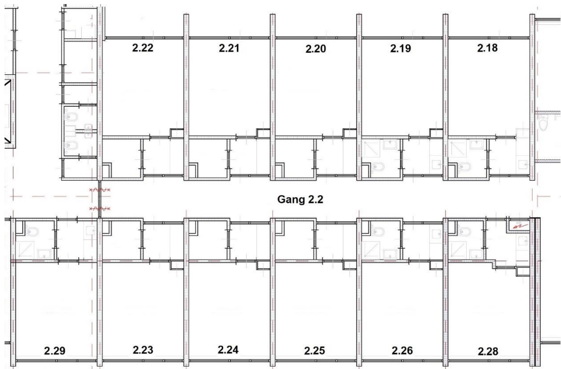
Figuur 3 Plattegrond tweede verdieping
