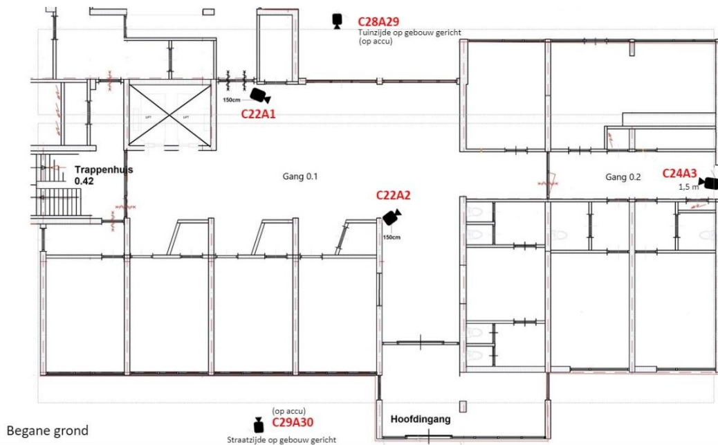
Figuur 5 Cameralocaties op de begane grond
