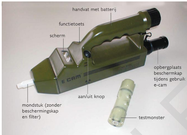
Figuur 8.8 De E-CAM
