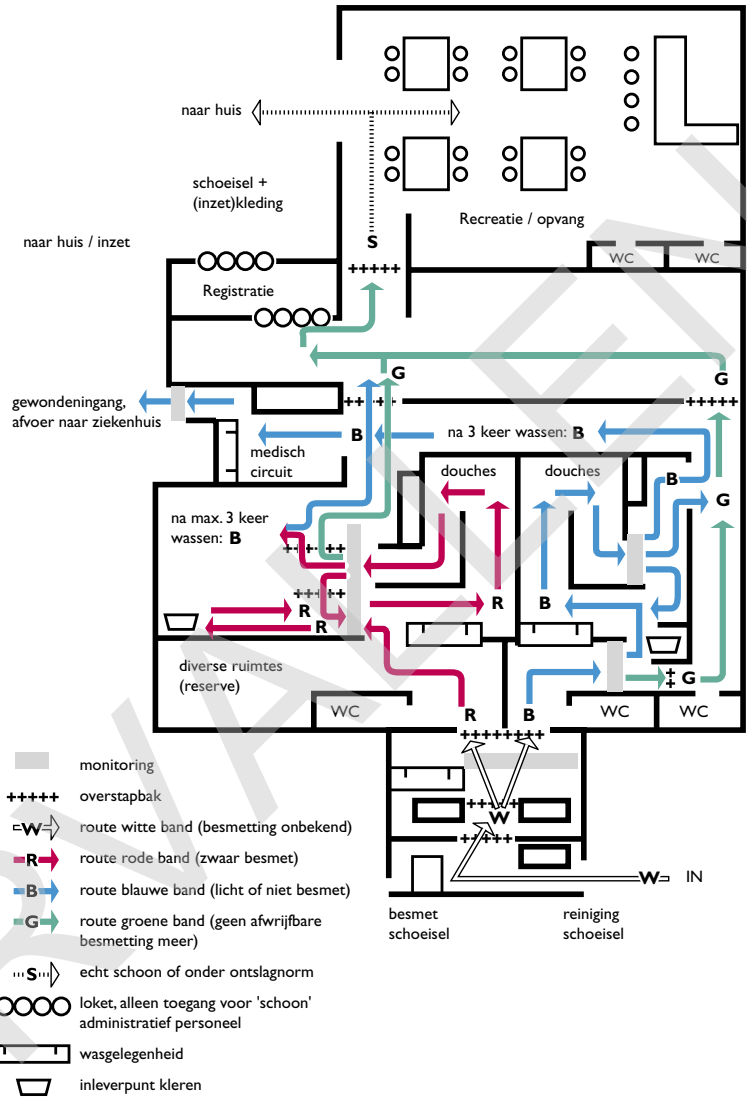
Figuur 6.9 Mogelijke indeling van ontmettingsruimte
