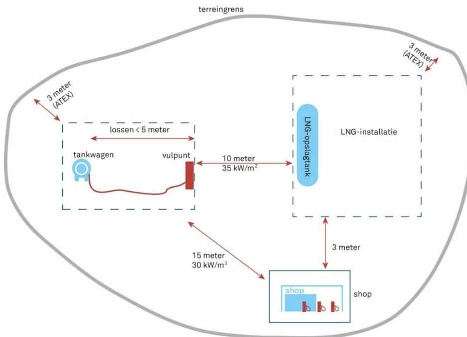
Afbeelding B.4 Een overzicht van de interne veiligheidsafstanden die gelden voor LNG-tankstations
