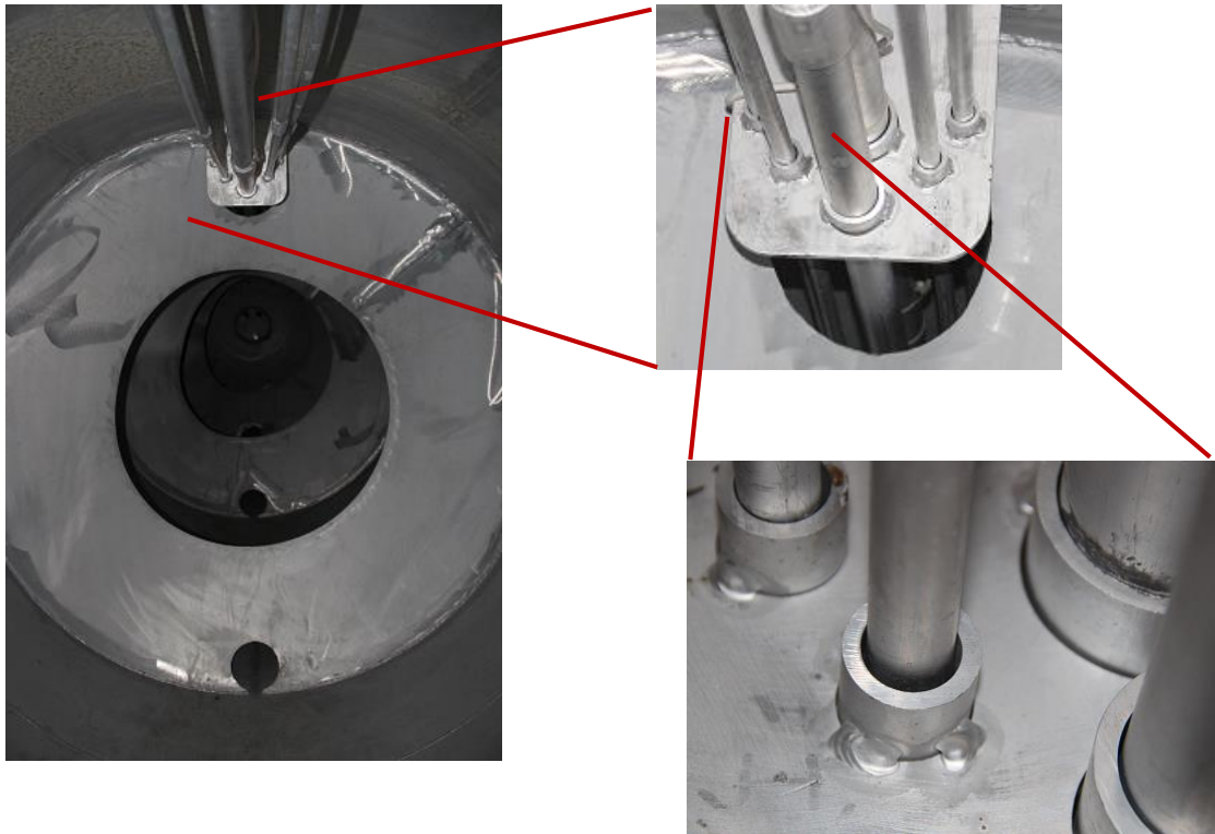
Afbeelding 5.12 Slingerschotten in de tank: links het slingerschot en rechts uitvergrotingen van de doorvoering van leidingen door de schotten
